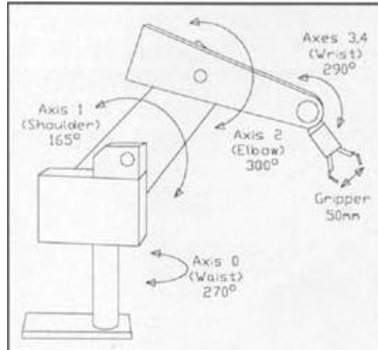
รูปที่ 3 การเคลื่อนไหวของแขนกล Gryphon
